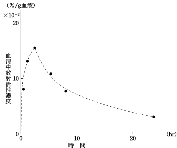
図VII-4. 14 C-ジソピラミドをラットに経口投与したときの血清中放射活性濃度の時間推移
