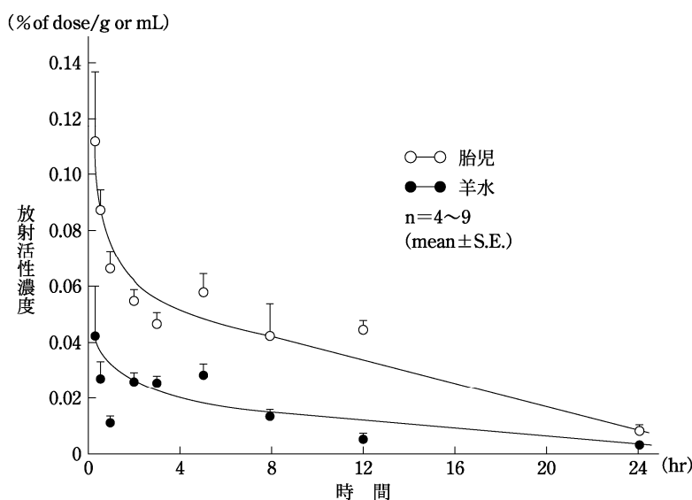
図VII-5. ^{14}\text{C} -ジソピラミドリン酸塩を妊娠ラットに静脈内投与したときの胎児及び羊水の放射活性の時間推移
